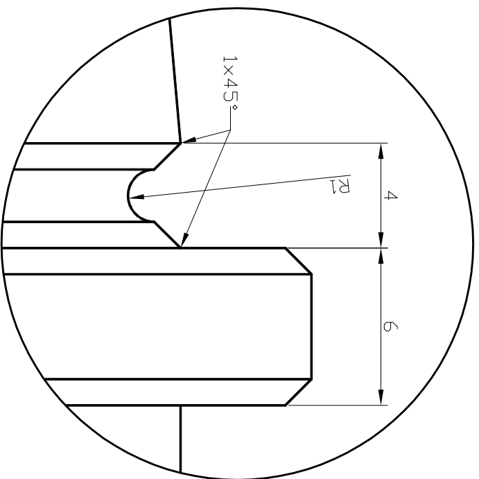
Szczegół A (5:1)
