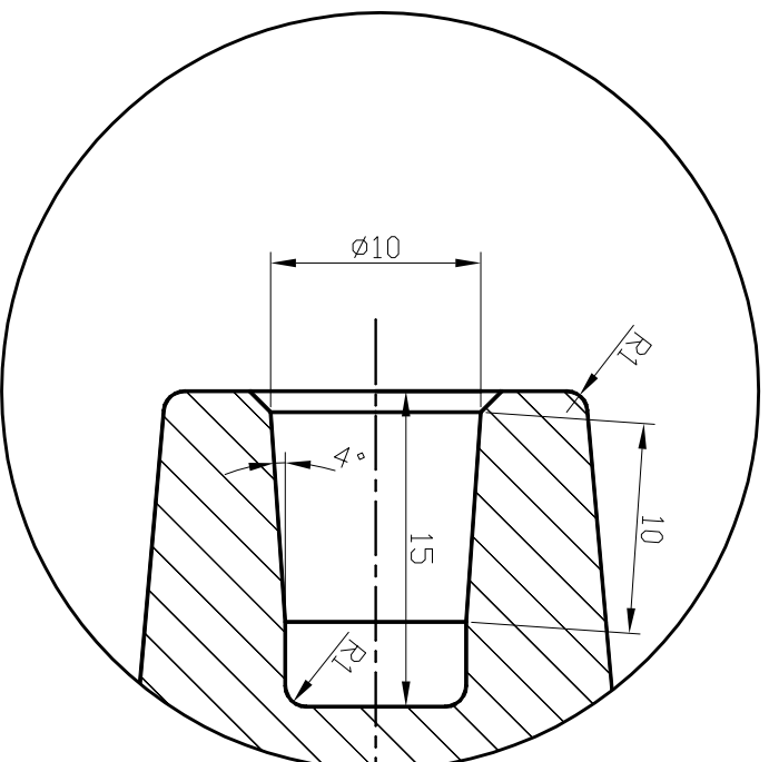
Szczegół B (2,5:1)
